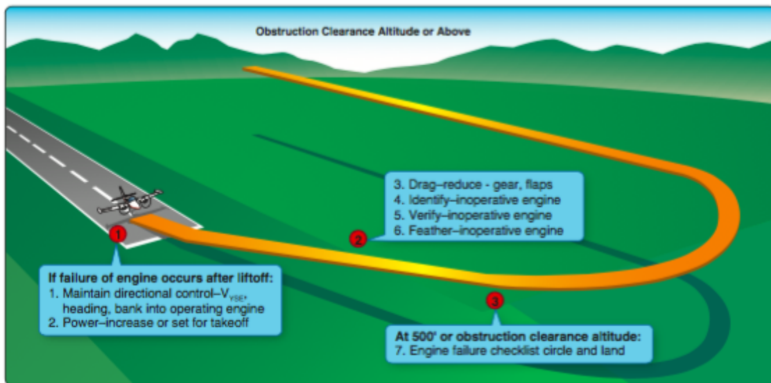
Figura 12-13. Performance adecuada de ascenso con tren retraído
