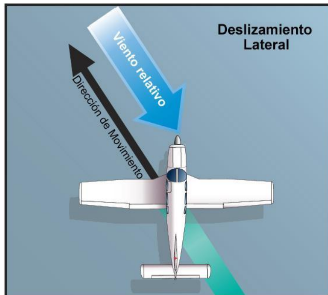
Figura 8-12. Deslizamiento lateral.
