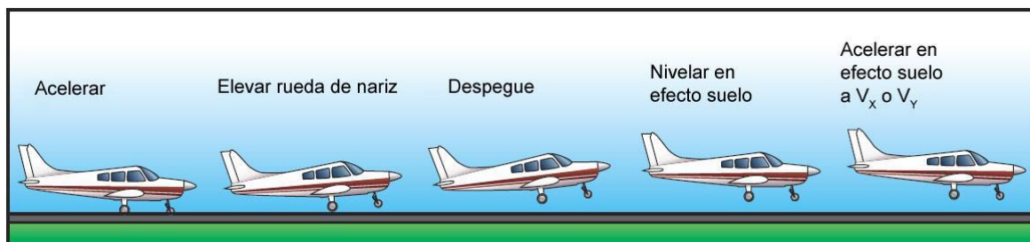
Figura 5-9. Despegue en campo blando.
