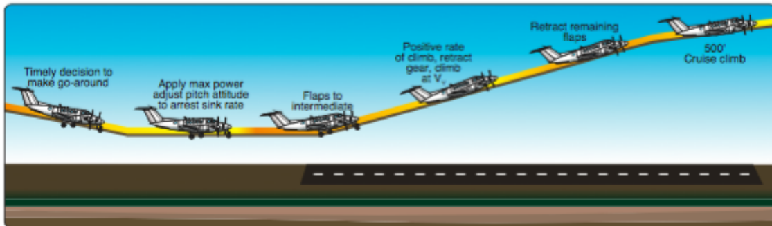
Figura 12-10 Procedimiento de escape
