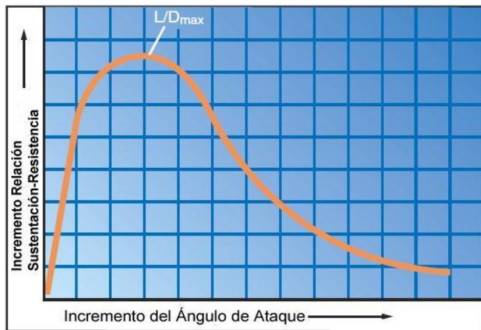
Figura 3-17. L/D MAX .
