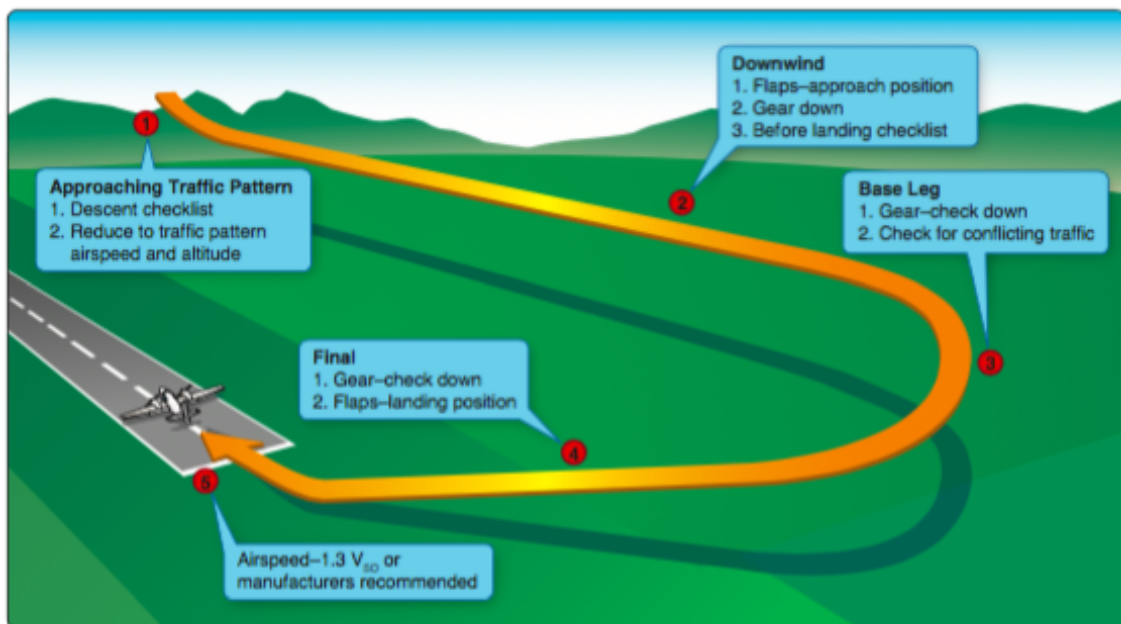
Figura 12-8. Aproximación y aterrizaje normal con un bimotor
