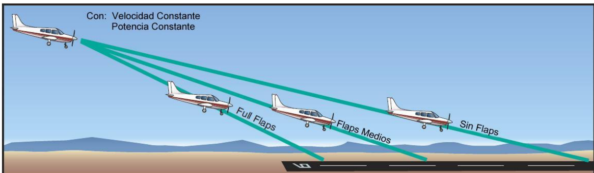
Figura 8-3. Efecto de los flaps en el punto de aterrizaje.
