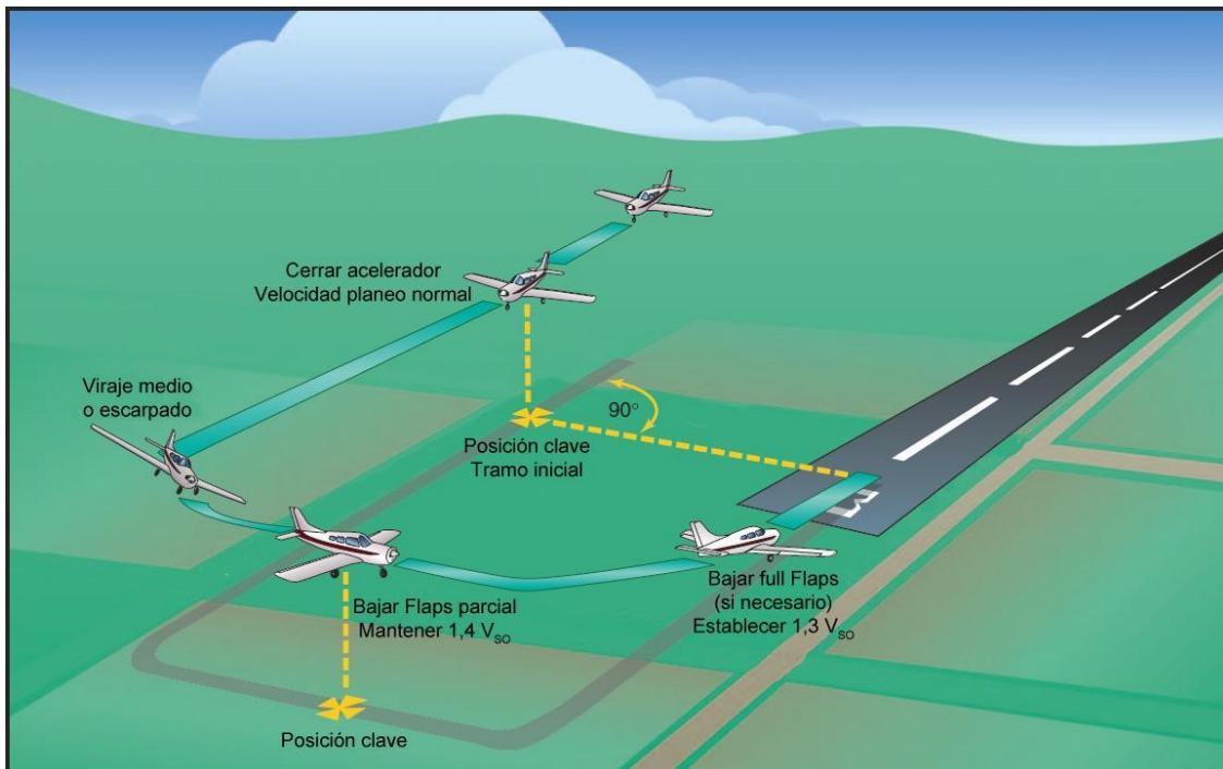
Figura 8-27. Aproximación sin potencia de 180°.
