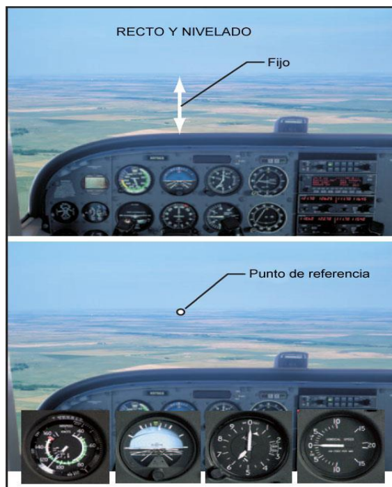
Figura 3-3. Referencia de nariz para vuelo recto y nivelado.
