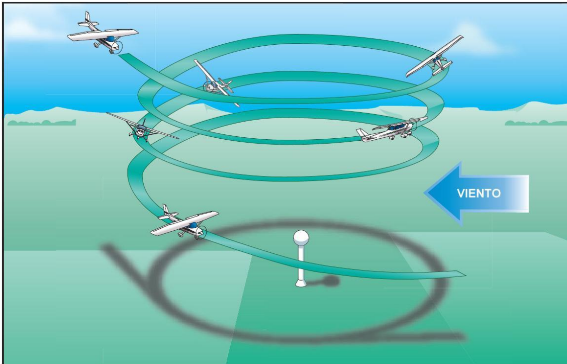
Figura 9-2. Espiral escarpada.
