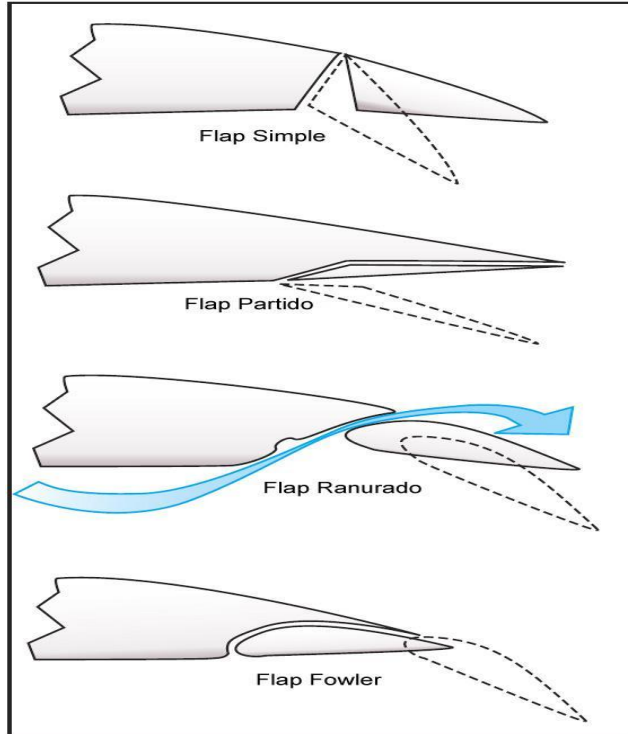
Figura 11-2. Cuatro tipos básicos de flaps.
