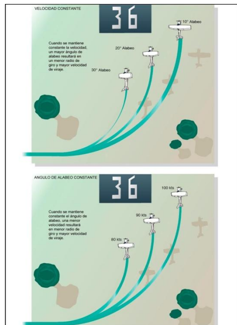
Figura 3-9. La velocidad y el ángulo de alabeo regulan el radio y velocidad del giro.
