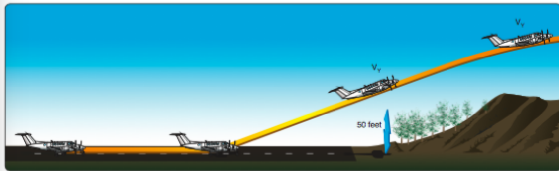
Figura 12-9. Despegue y ascenso en campo corto.
