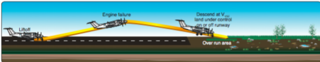
Figura 12-12. Falla de motor en el despegue. Performance inadecuada de ascenso.
