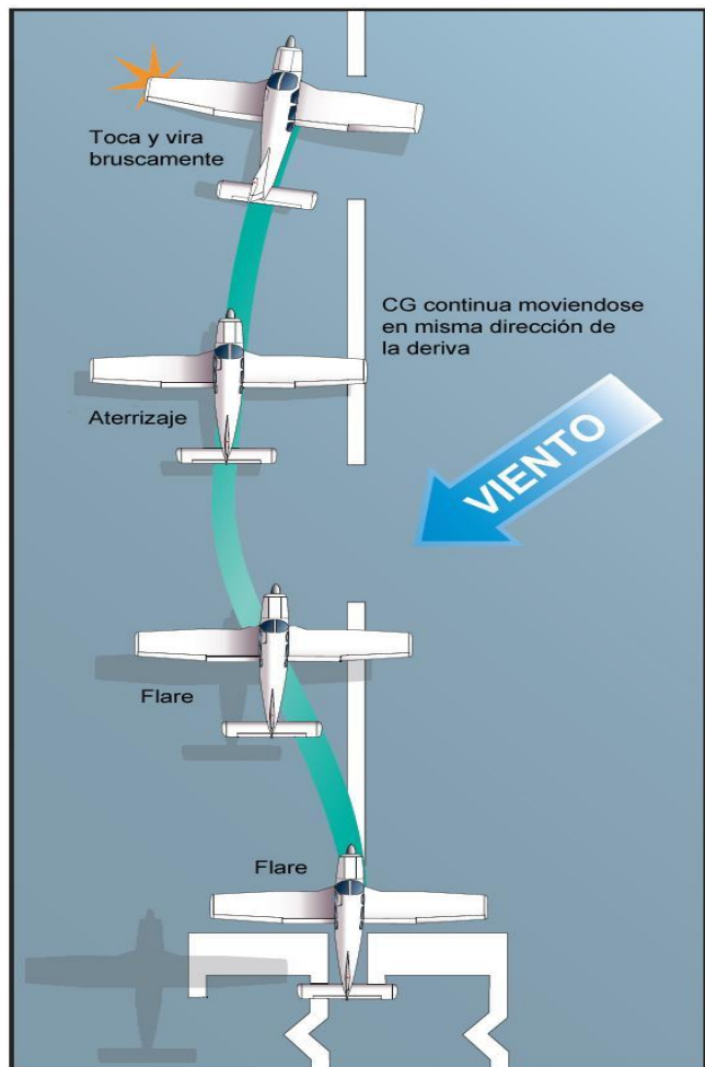
Figura 8-39. Inicio de un trompo.
