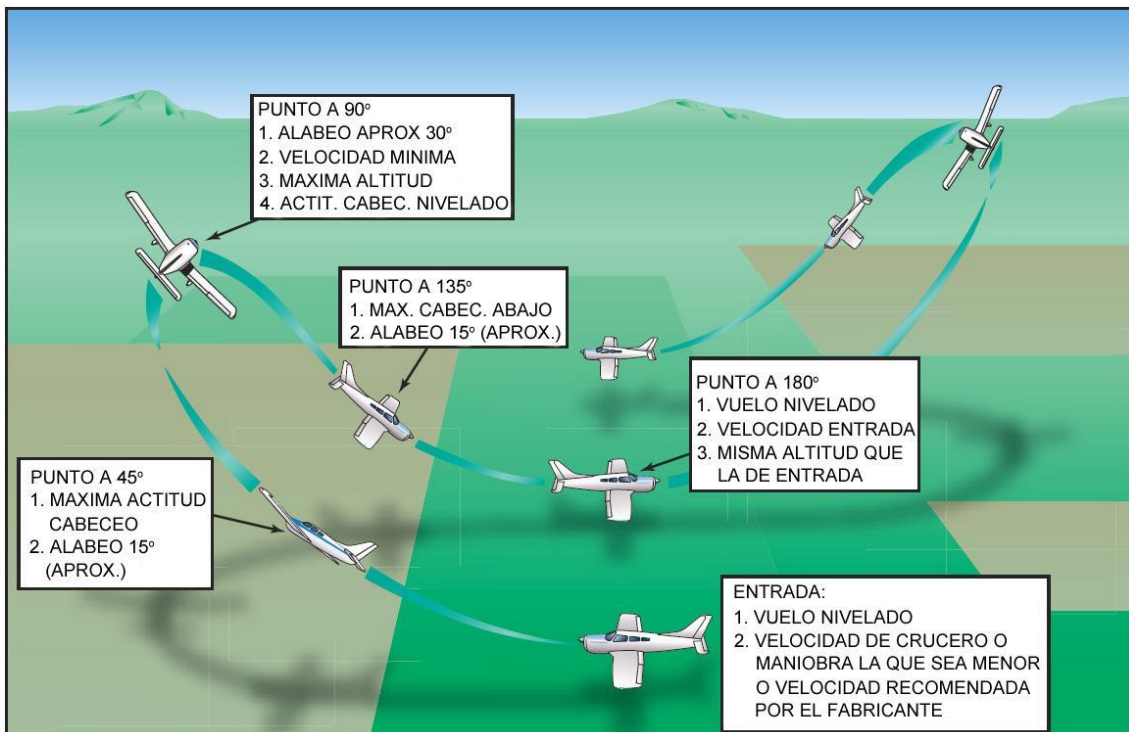
Figura 9-5. Ocho perezoso.
