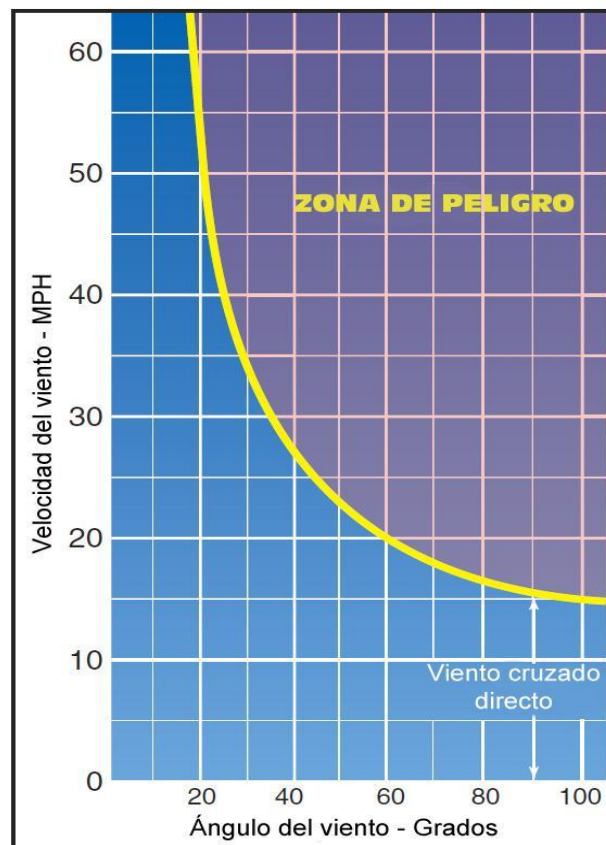
Figura 8-18. Tabla de viento cruzado.
