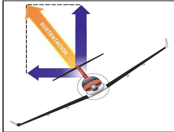
Figura 3-6. El cambio en la sustentación produce que el avión viere.
