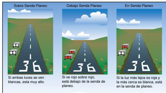
Figura 10-5. VASI.
