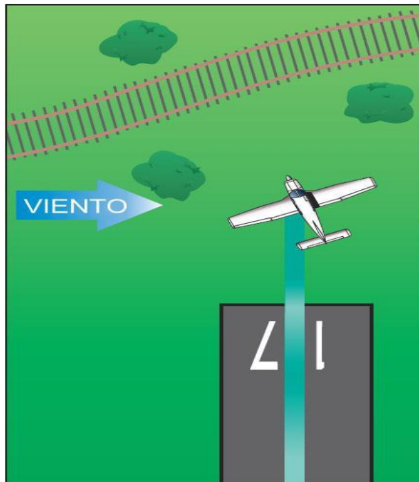
Figura 5-5. Trayectoria de ascenso con viento cruzado.
