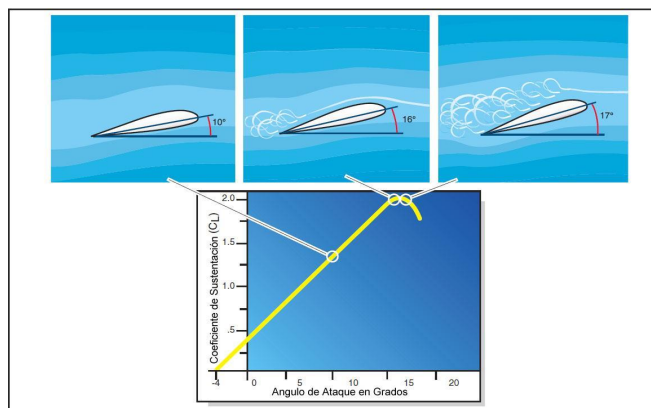
Figura 4-2. Ángulo de ataque crítico y pérdida.
